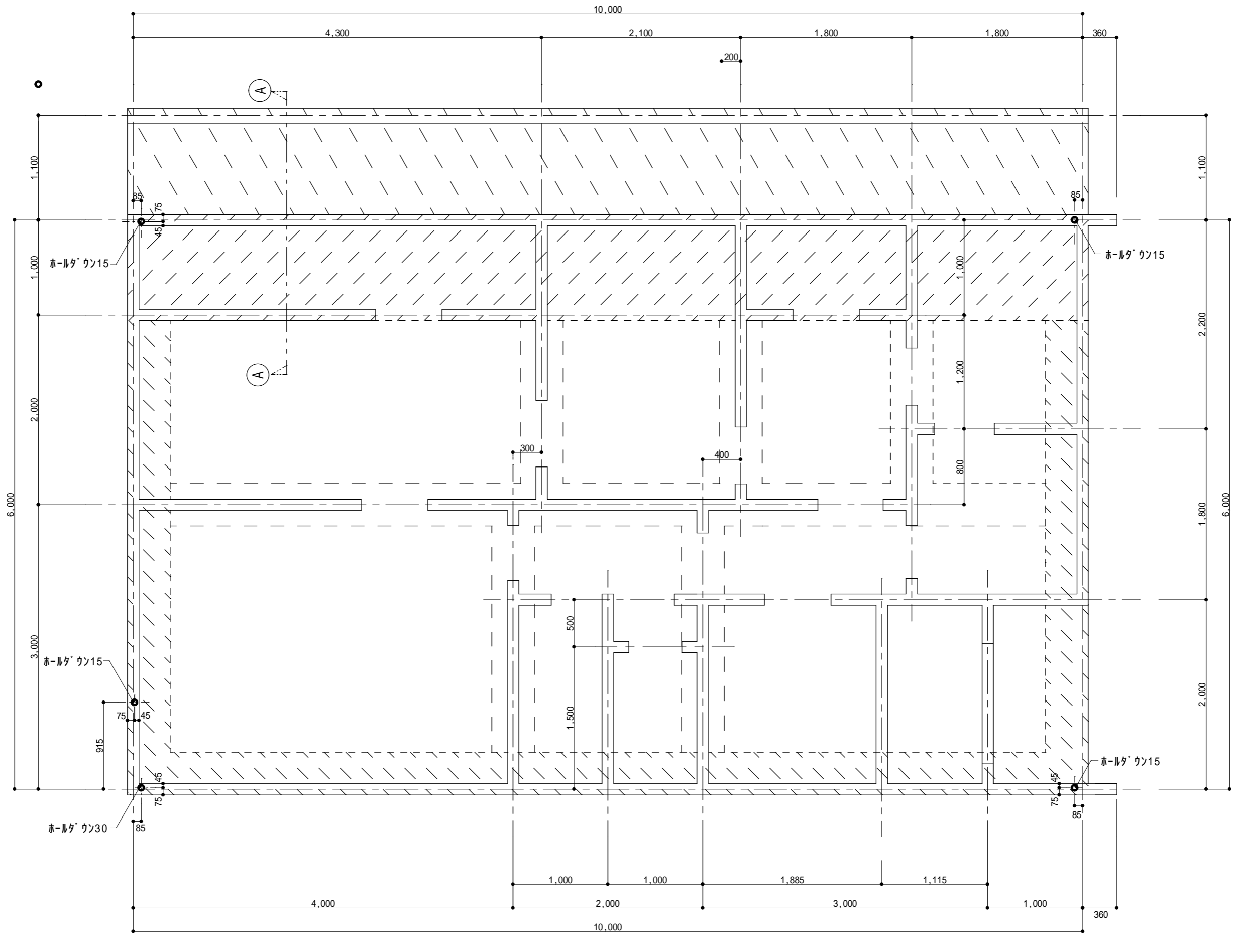
基礎伏図 S = 1:40
